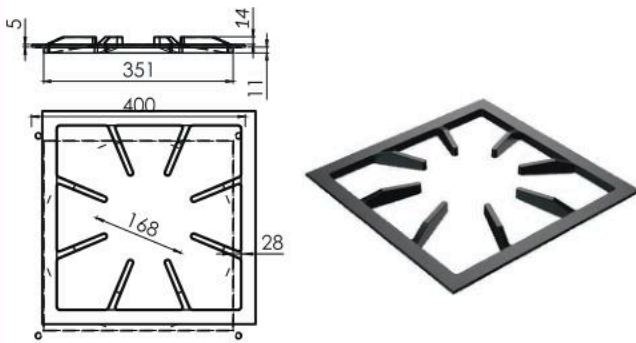
GRELHA 8 HASTES 40 X 40 GSO CÓD 91.790
