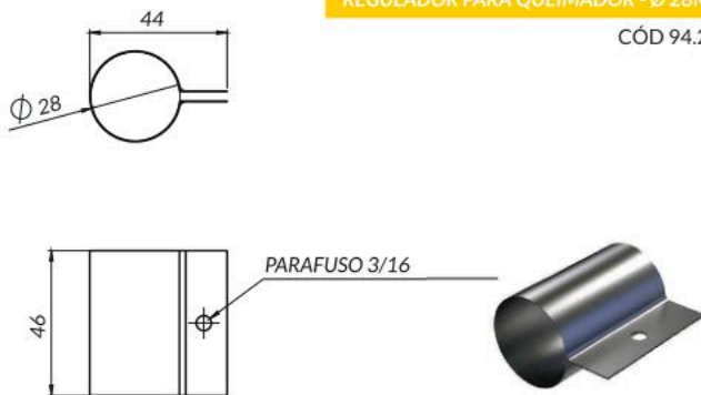
REGULADOR PARA QUEIMADOR - Ø 28MM
